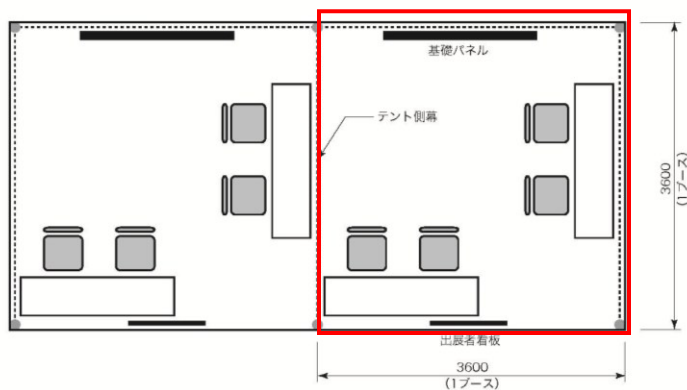
平面図
