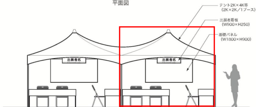
正面図
